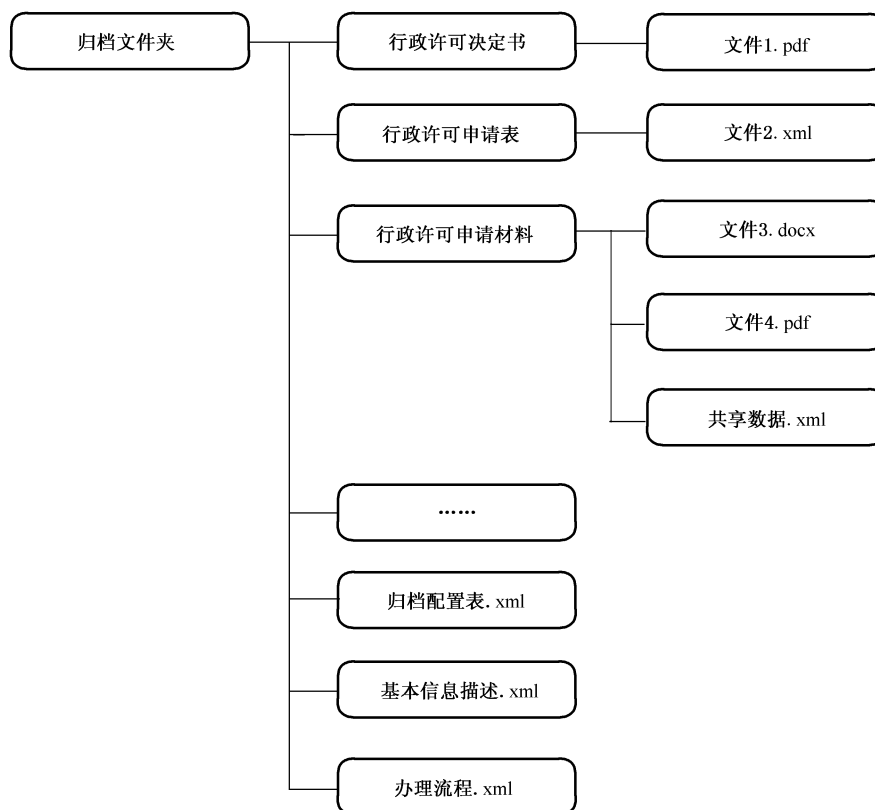
图 C.1 归档信息包的一般结构示例
