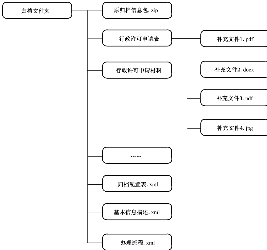
图 D.1 归档信息包的嵌套结构示例
